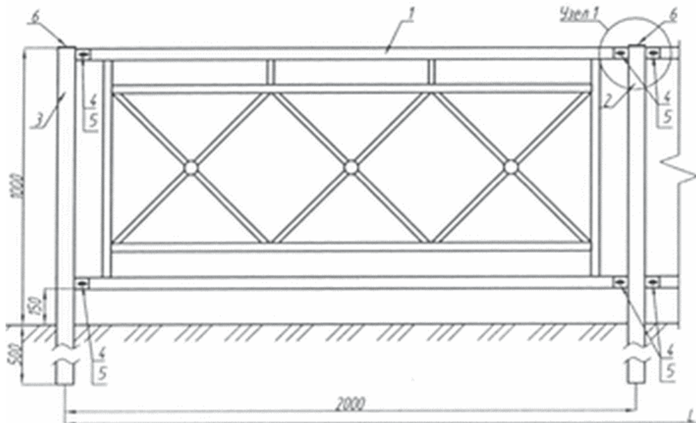
Тип 2: магистральное пешеходное ограждение безопасности
